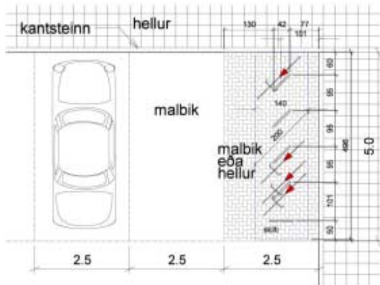
Hjólagrindur 45° grunnmynd 1:100
