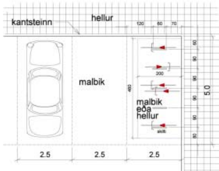
Hjólagrindur 90° grunnmynd 1:100
